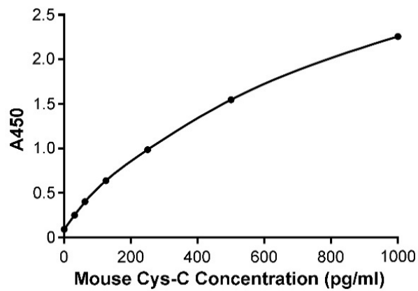
图3. Mouse Cys-C ELISA Kit的标准曲线。实测数据会因实验条件、检测仪器等的不同而存在差异，图中数据仅供参考。
